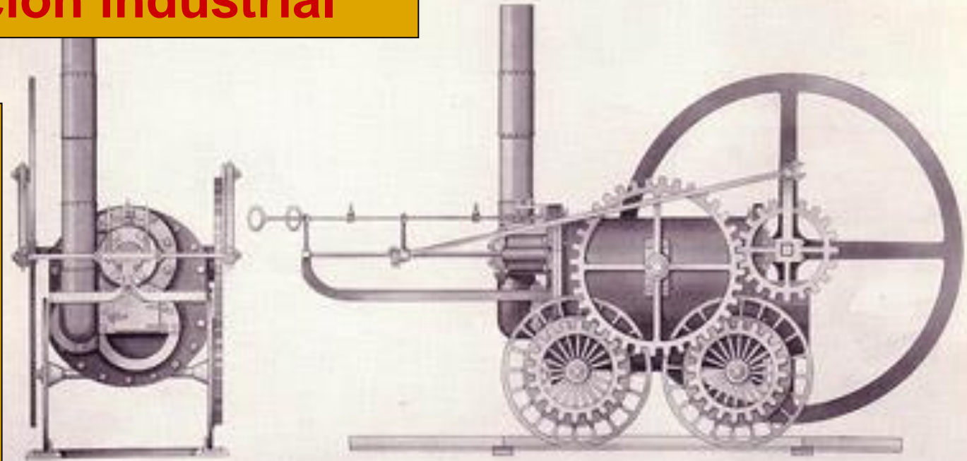
Locomotora de vapor diseñada por Richard Trevithick en 1804 en Inglaterra
